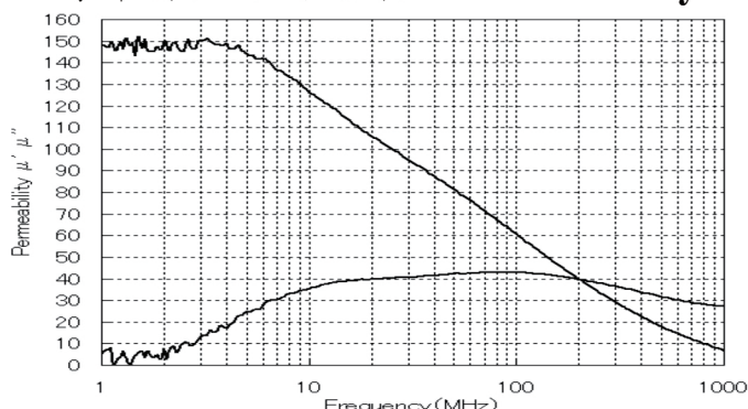
磁导率特性曲线 (图) Permeability
