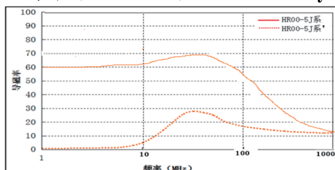
磁导率特性曲线 (图) Permeability
